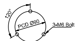
Stud Mount Hole Layout
