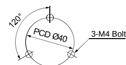
Stud Mount Hole Layout
